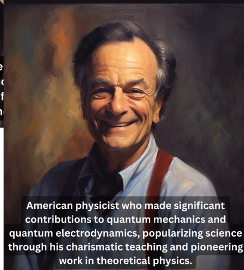
Richard Feynman
